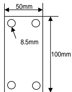
取付金具
